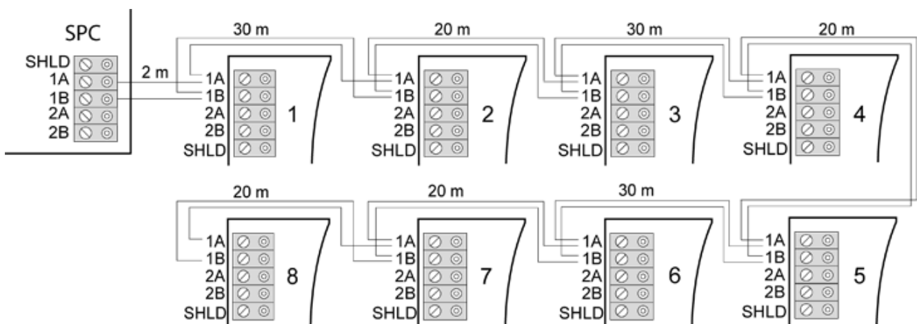
Multidrop-koppling
