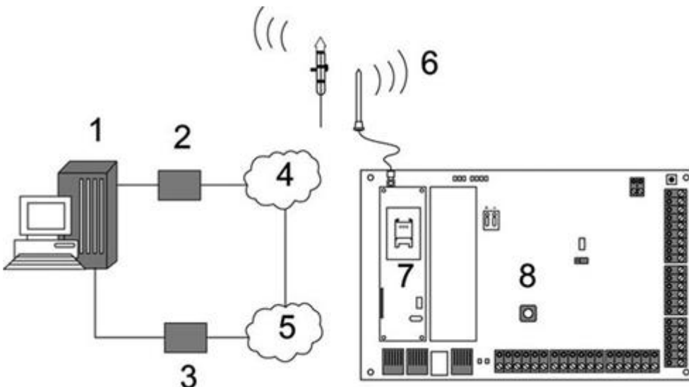
GSM-anlutning
