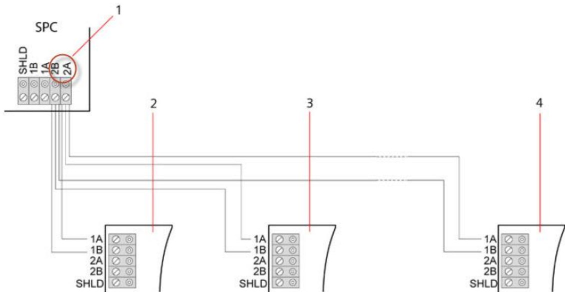
Stjärnkonfiguration 2
