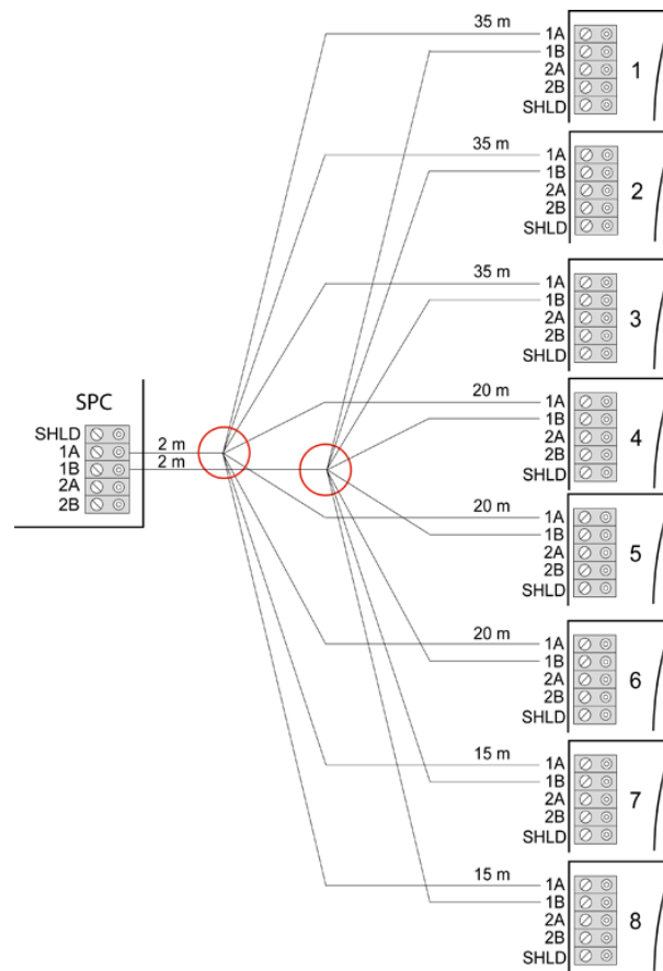
Stjärnkoppling
